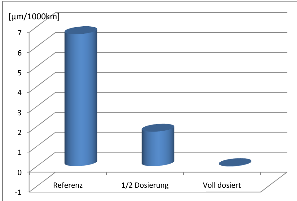
ABBILDUNG 5: VERSCHLEIßRATEN NACH DOSIERUNG
