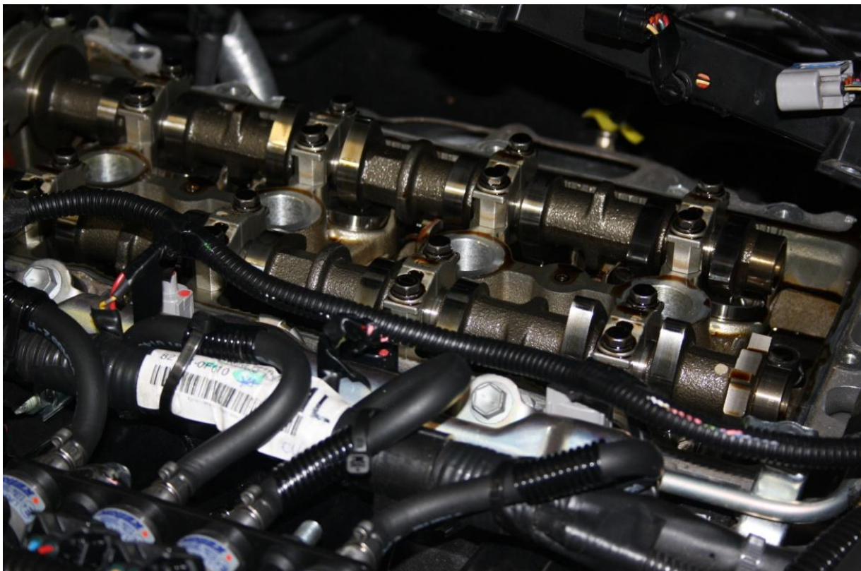
ABBILDUNG 1: VENTILTRIEB DES VERSUCHSFahrZEUGES
