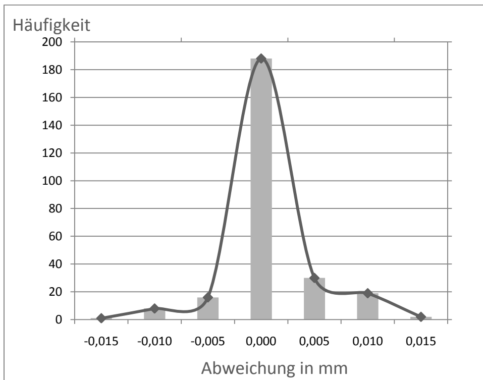
ABBILDUNG 6: HÄUFIGKEITSVERTEILUNG DER MESSABWEICHUNGEN
