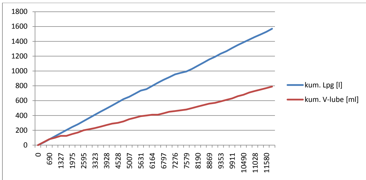
ABBILDUNG 3: DOSIERUNG / KOMMULIERTER VERBRAUCH
