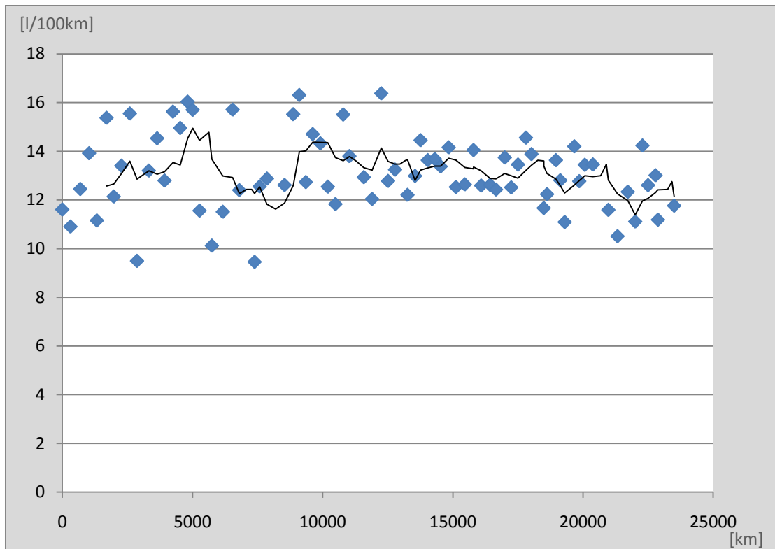
ABBILDUNG 7: GASVERBRAUCH PRO 100KM
