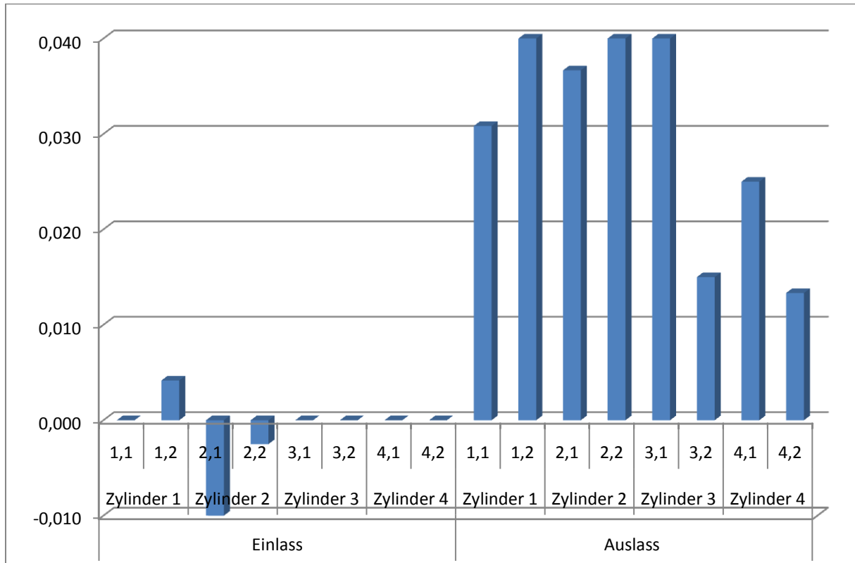
ABBILDUNG 2: ALLE VENTILVERSCHLEIß IN REINEN LPG-BETRIEB
