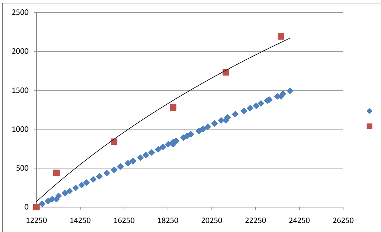
ABBILDUNG 4: DOSIERUNG / KUMULIERTER VERBRAUCH NACH HERSTELLER MINDESTANGABE
